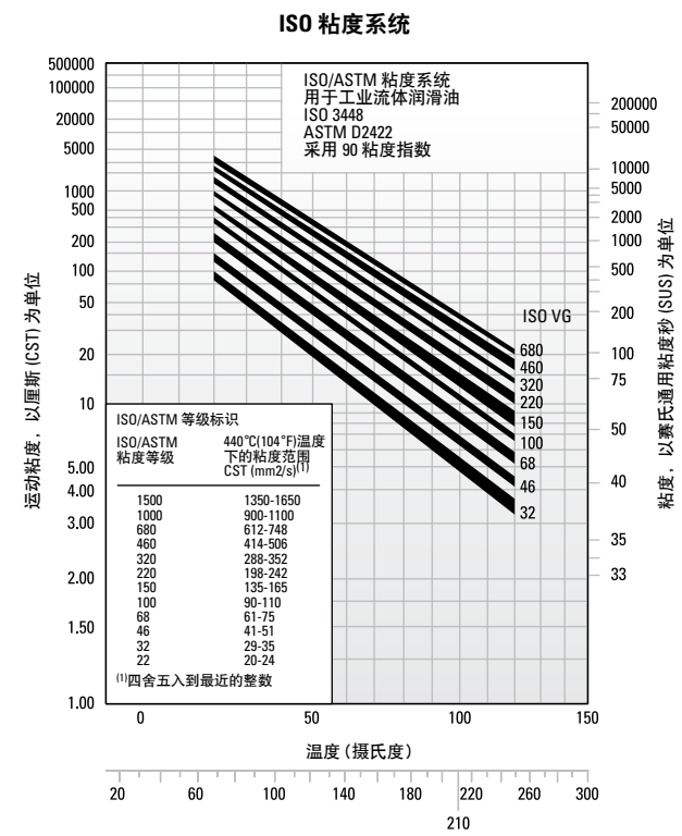
图 22. 工业润滑油粘度等级系统
