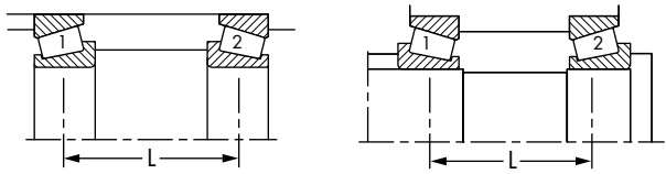
图 16. 面对面与背对背安装
