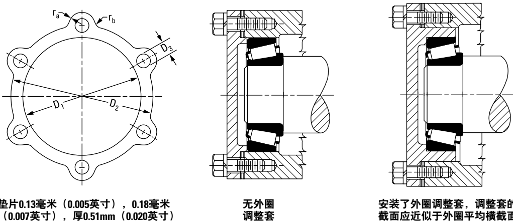
图 57. 外圈垫片
